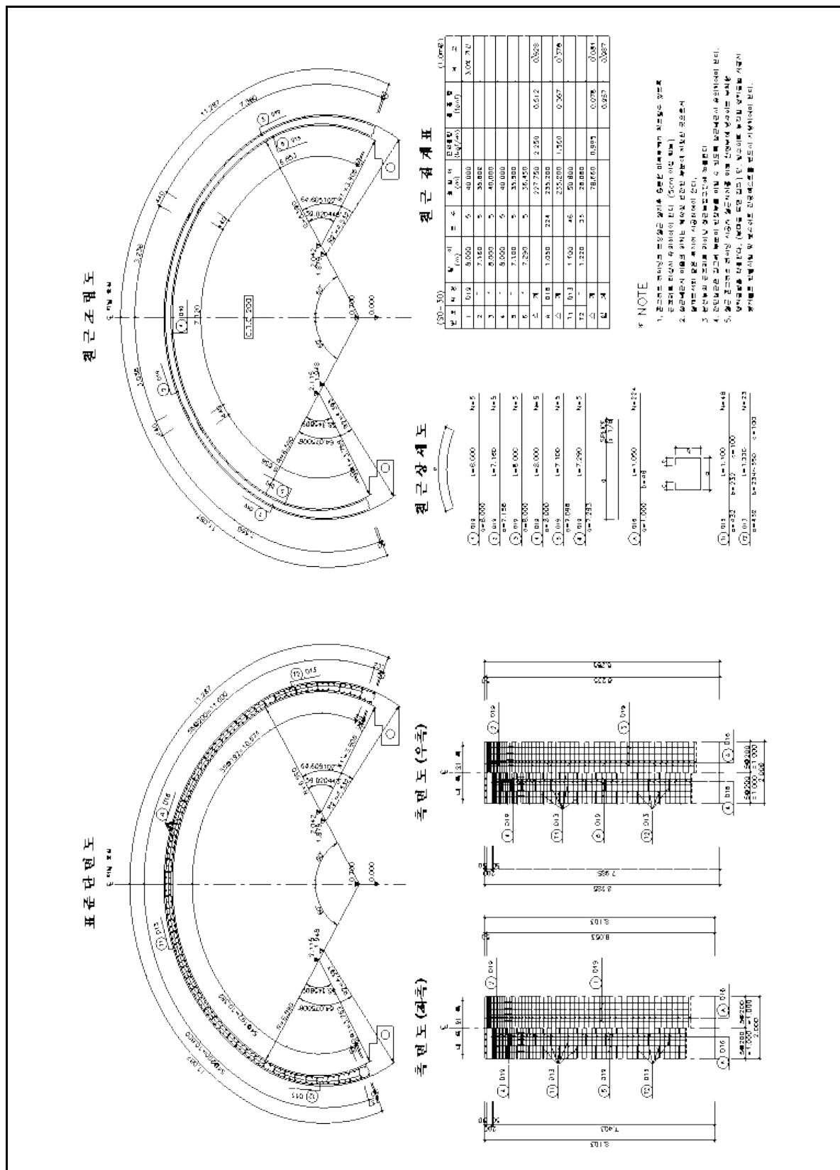
【그림 1.4】 군자2터널(서울) 콘크리트 라이닝 철근 보강도
